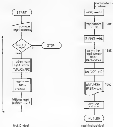
Afb. 4-1 Flowcharts van BASIC- en machinetaalprogramma
